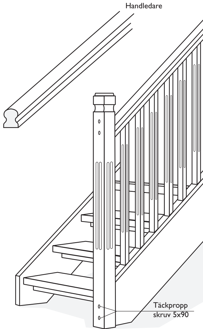
Handledare 60x70 (utan list) Överliggare 60x70 (med list)
